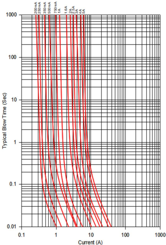
5J Time-Current Characteristic Curves 平均時間 - 電流曲線
